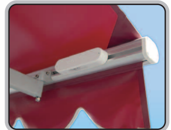
■振動センサー (アルタス専用オプション) 風によるオーニングの揺れを感知してキャンバスを巻き取る装置。強風対策に。
