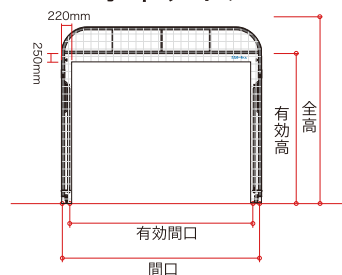
水平タイプ
