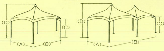
外寸法図
