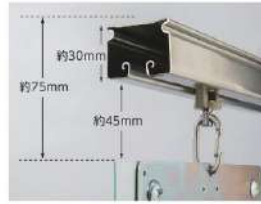
● ステンレス カーテンレール (20w)
