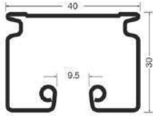
● ステンレス カーテンレール (旧10w)
