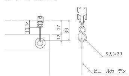
サンリブ19+Sカン29
