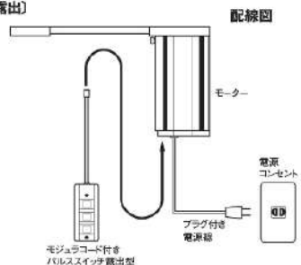
配線図
