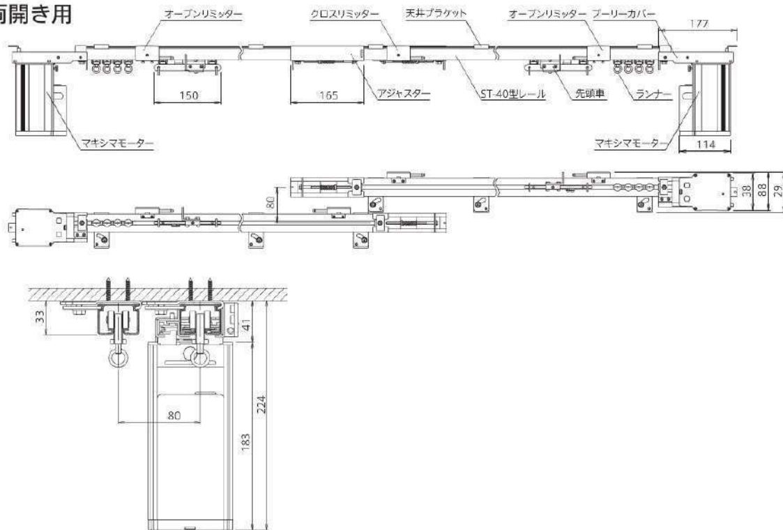
マキシマ取付寸法図 (ST-40)
