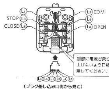
結線図
