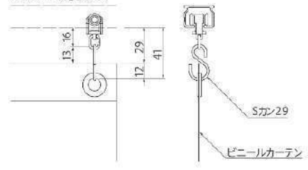
サンリブ19+Sカン29
