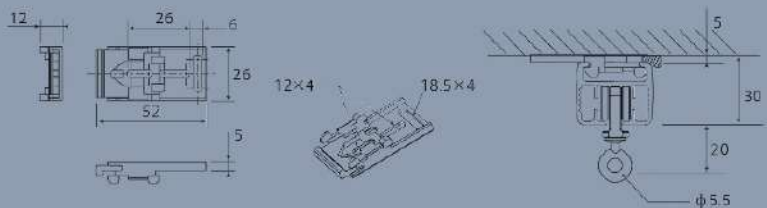
ブラケット寸法図
