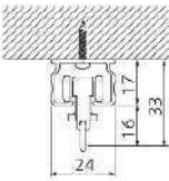
天井直付
