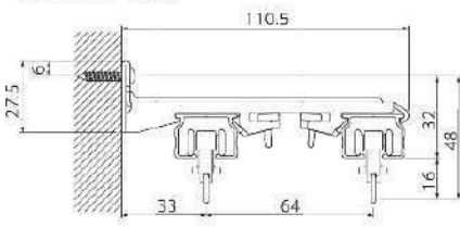
ダブルブラケット付 (ブラケット幅=22mm)
