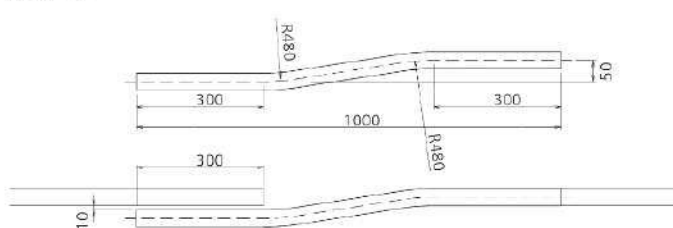
交叉レール
