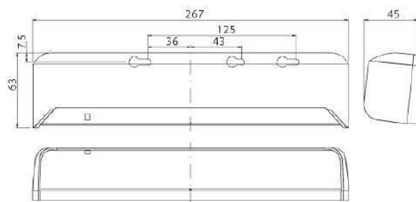
赤外線センサー外観図
