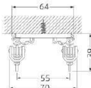
天井ダブルブラケット付 (ブラケット幅=20mm)
