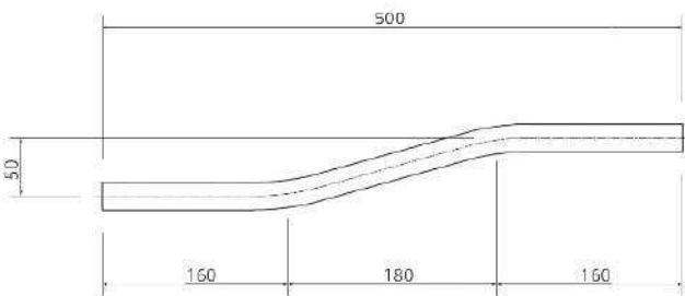
交叉レール
