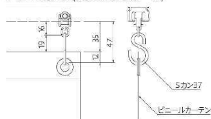
サンリブ19+Sカン37(ステンレス・スチール)
