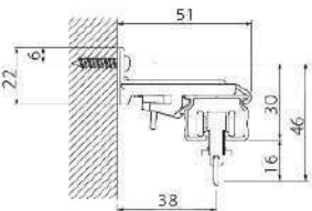
シングルブラケット付 (ブラケット幅=19mm)
