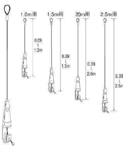
Nスライドハンガー-YF-20/YF-30
