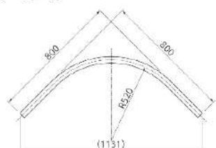
カーブレール
