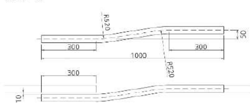
交叉レール
