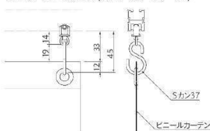
サンリブ19+Sカン37(ステンレス・スチール)
