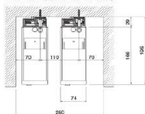
■ダブル付(天井ブラケット使用)
