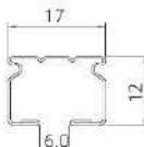
ステンレス
