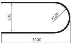
U 字型カーブ 450R
