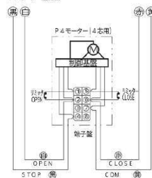
P4 モーター配線図
