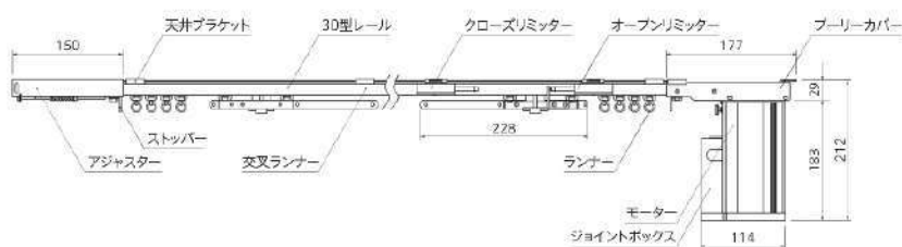
■天井ブラケット付
