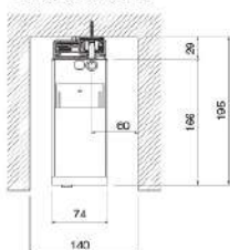
■天井ブラケット付
