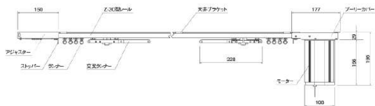
■天井ブラケット付
