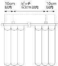
ブラケットの取り付けピッチとカーテン適正重量
