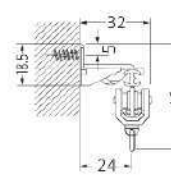
シングルブラケット付 (ブラケット幅=18mm)
