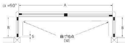
U字形カーブレール (シングル付)
