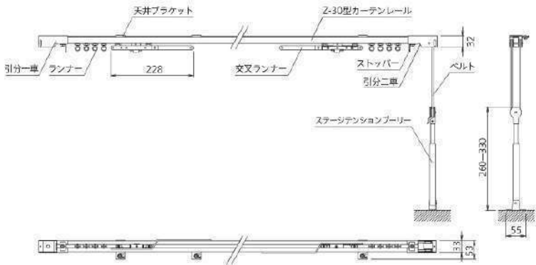
30 型紐引きカーテンレール寸法図
