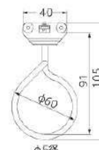
点滴ランナー(事故防止タイプ)
