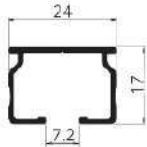
レール断面図 (mm)
