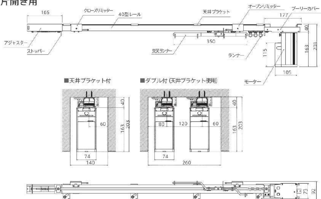
ニューII型取付寸法図 (Z-40)
