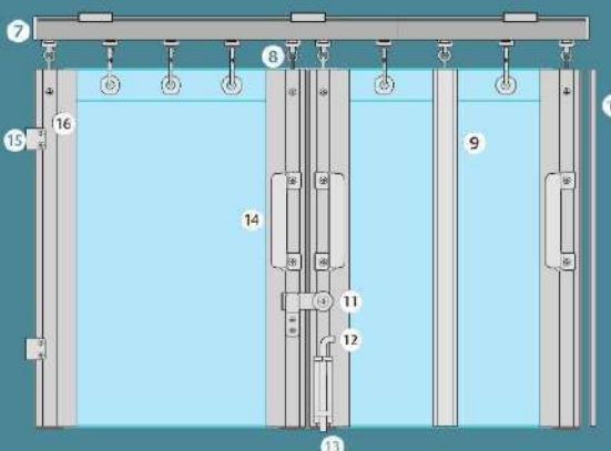
⑪両開きロック金具
