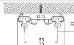
ワンタッチ天井ダブルブラケット付 (ブラケット幅=20mm)
