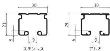
レール断面図
