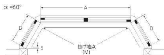
台形カーブレール (シングル付)
