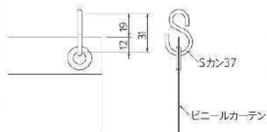
Sカン37(ステンレス・スチール)
