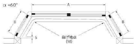
台形カーブレール (ダブル付)
