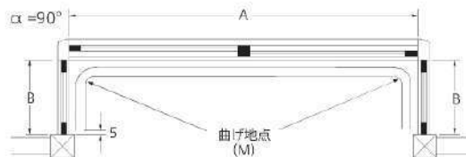
U字形カーブレール (ダブル付)
