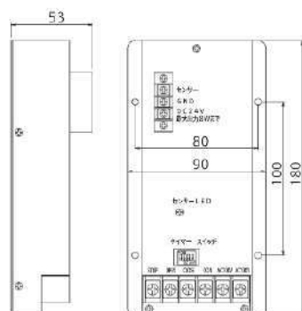
カーテン制御ボックス外観図
