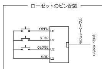
グリディア配線図 (有線)
