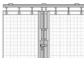
両開き間仕切フレーム2本タイプ
