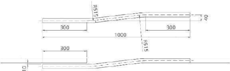
交叉レール
