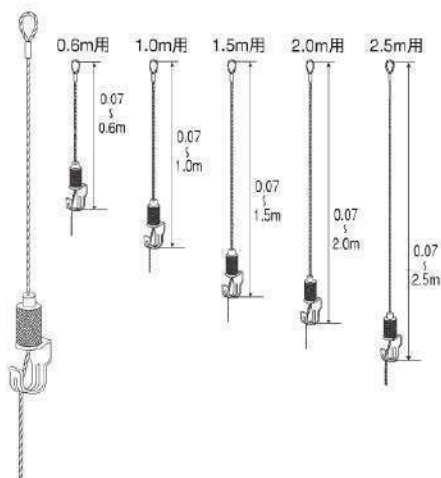
Nスライドハンガー-SH-10
