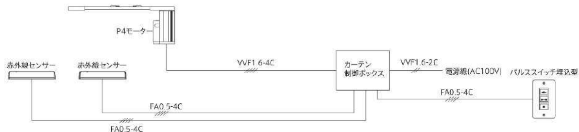
P4 モーター配線図
