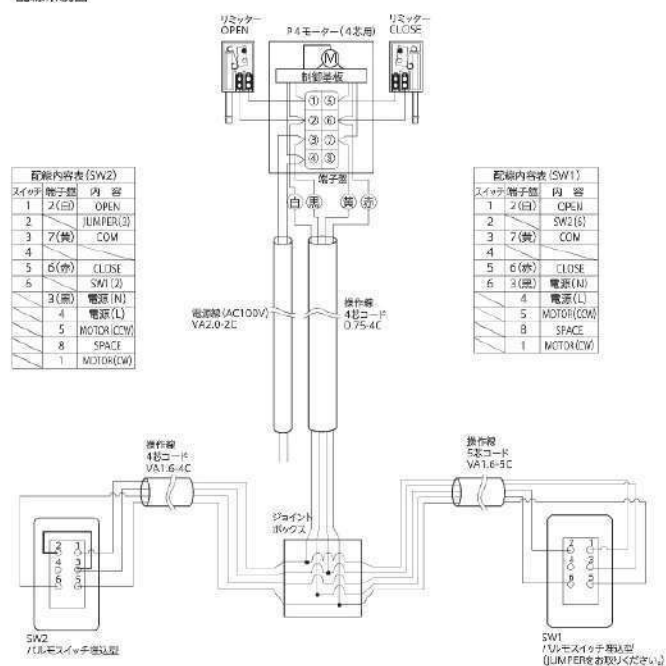
配線系統圖
