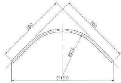
カーブレール
