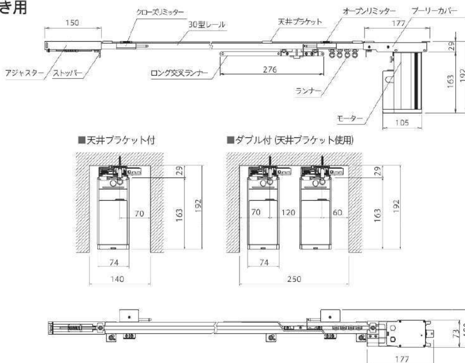
ニューII型取付寸法図 (Z-30)
