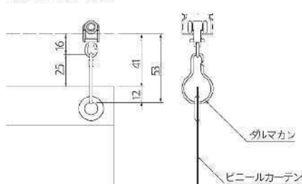
N-24+ダルマカン
