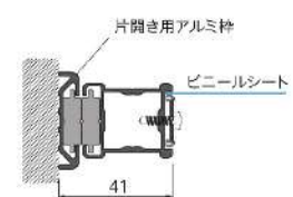
片開き納まり図
