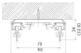
ワンタッチ天井ダブルブラケット (70mm)
