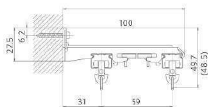
ワンタッチダブルブラケット (59mm)
