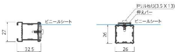
サイドフレーム ライト
