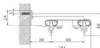
ワンタッチ正面ダブルブラケット 55 付 (ブラケット幅=20mm)
