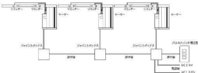
P6 モーター (DC2.4V) 一斉操作パルススイッチ (埋込)
