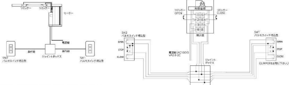
P4モーター (4芯AC付) 両面操作パルモスイッチ [埋込]
