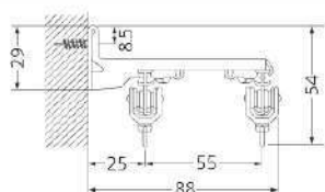
ダブルブラケット付 (ブラケット幅=20mm)
