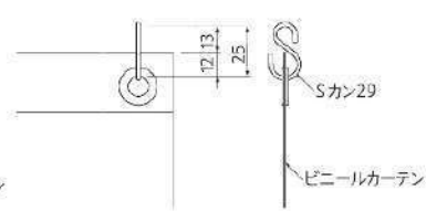
Sカン29(スチール)
