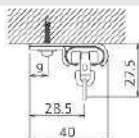
天井シングルブラケット付 (ブラケット幅=13mm)
