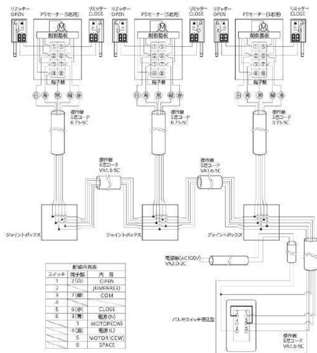
配線系統図
