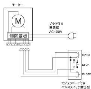
ミディアム配線図
