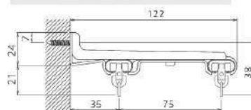
ワンタッチ正面ダブルブラケット 75 付 (ブラケット幅=22mm)
