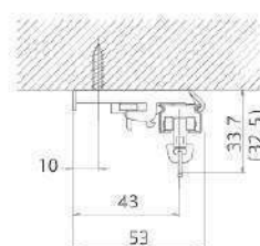
ワンタッチ天井シングルブラケット
