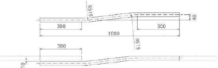
交叉レール
