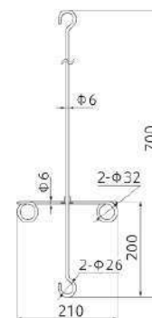
十字ハンガー
