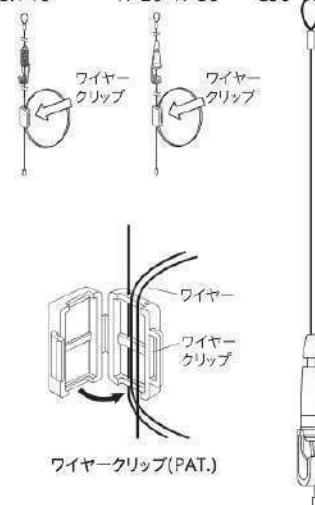
Nスライド ハンガー SH-10
