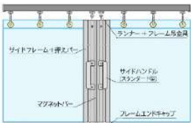
セット構成 TYPE 1
