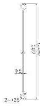
ストレートハンガー
