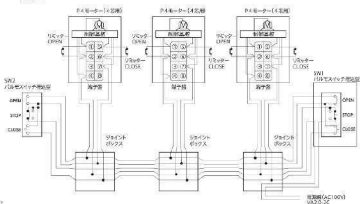
配線図
