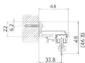
ワンタッチシングルブラケット
