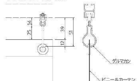
サンリブ19+ダルマカン
