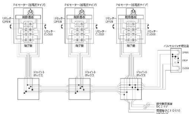
配線図
