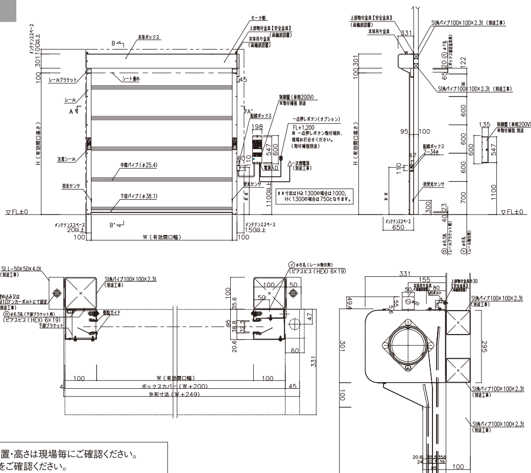
RB-1Ta 納まり図
