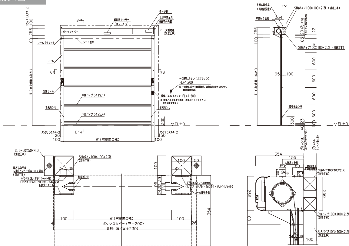
RB-1 納まり図
